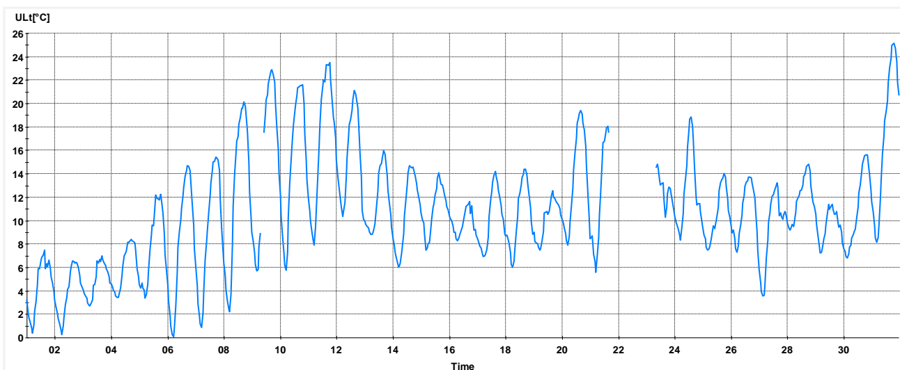
ULt[°C] Monthly Report Terveyskeskus 05.2011 Interval 1 Hour
