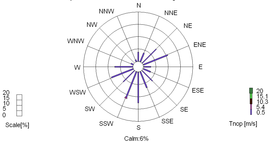
Monthly Wind Rose Terveyskeskus toukokuu 2011 Station:Terveyskeskus Avg:1 Hour
