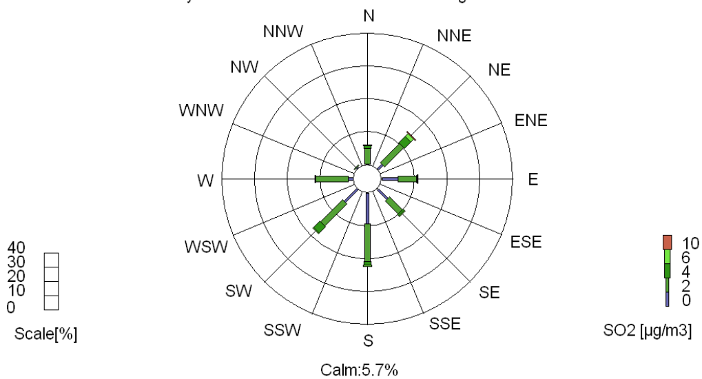
Monthly Pollution Rose Terveyskeskus toukokuu 2011 Station:Terveyskeskus Avg:1 Hour
