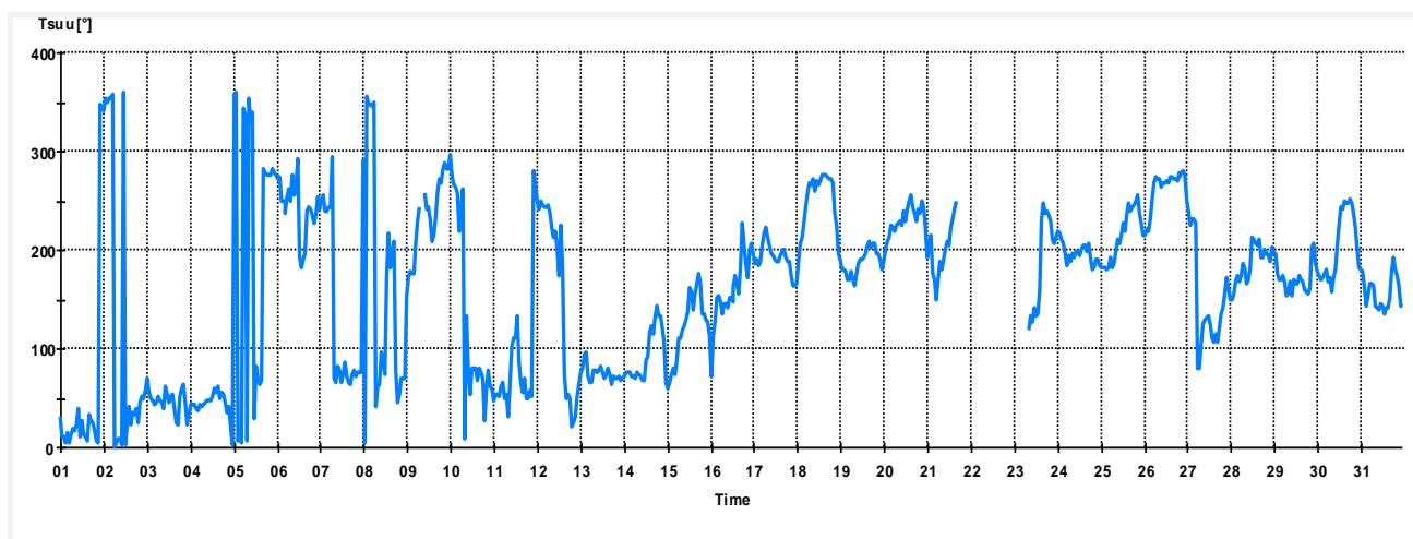
Tnop[m/s] Monthly Report Terveyskeskus 05.2011 Interval 1 Hour
