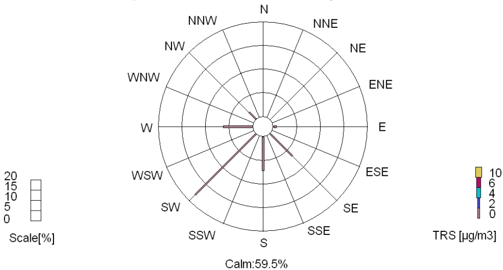
Monthly Pollution Rose Tekonurmi marraskuu 2011 Station:Tekonurmi Avg:1 Hour
