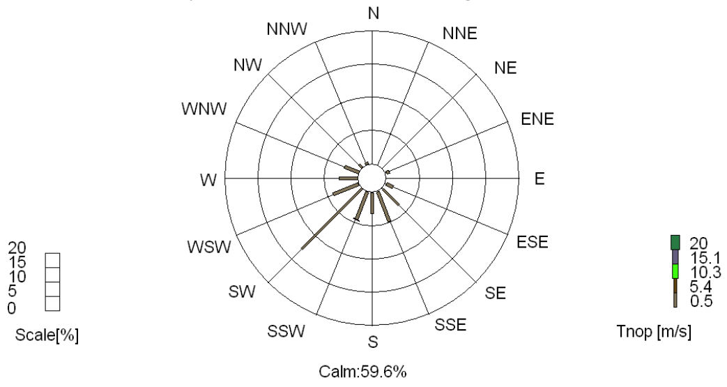
Monthly Wind Rose Terveyskeskus marraskuu 2011 Station:Terveyskeskus Avg:1 Hour
