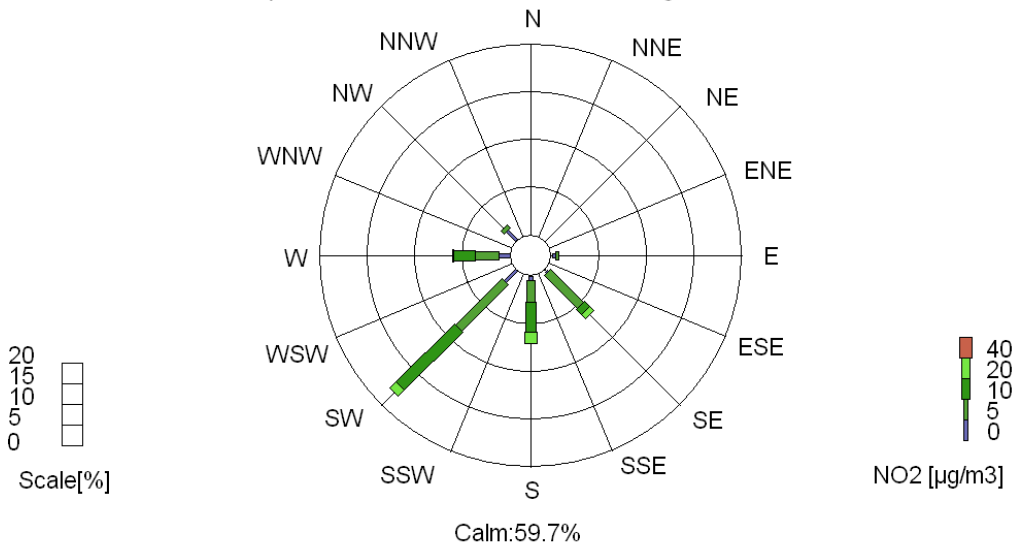
Monthly Pollution Rose Terveyskeskus marraskuu 2011 Station:Terveyskeskus Avg:1 Hour
