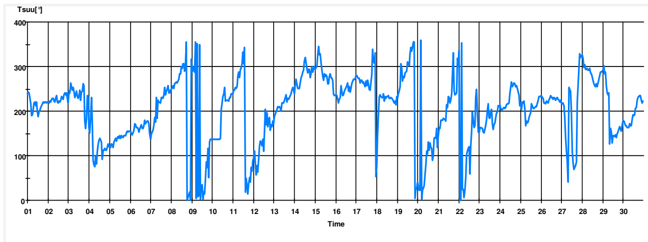
Tsuu[°] Monthly Report Terveyskeskus 11.2011 Interval 1 Hour
