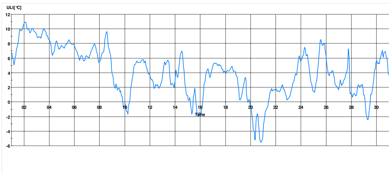
ULt[°C] Monthly Report Terveyskeskus 11.2011 Interval 1 Hour
