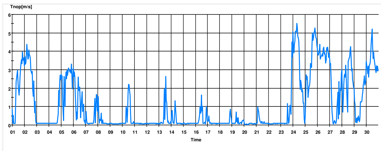
Tnop[m/s] Monthly Report Terveyskeskus 11.2011 Interval 1 Hour
