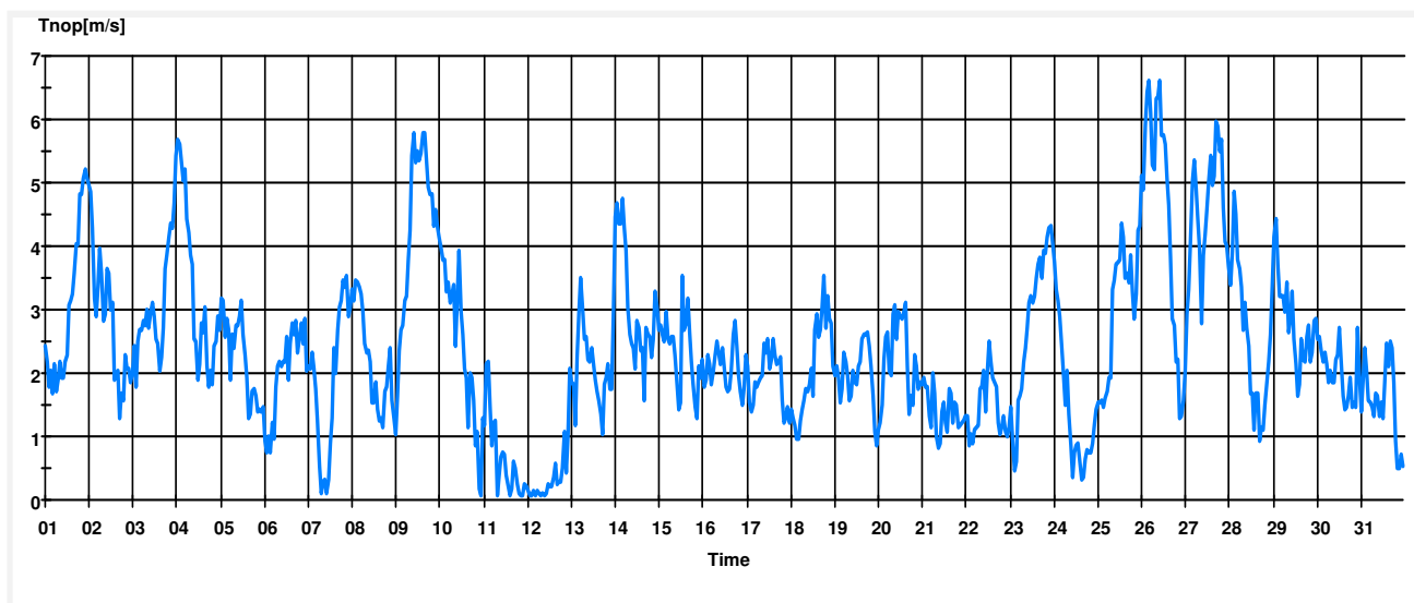
Tnop[m/s] Monthly Report Terveyskeskus 12.2011 Interval 1 Hour
