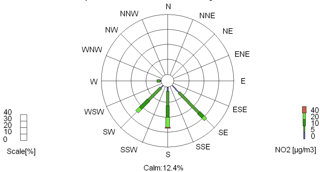
Monthly Pollution Rose Terveyskeskus joulukuu 2011 Station:Terveyskeskus Avg:1 Hour
