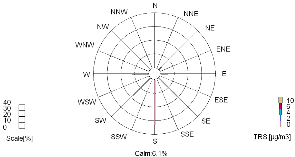
Monthly Pollution Rose Terveyskeskus joulukuu 2011 Station:Terveyskeskus Avg:1 Hour
