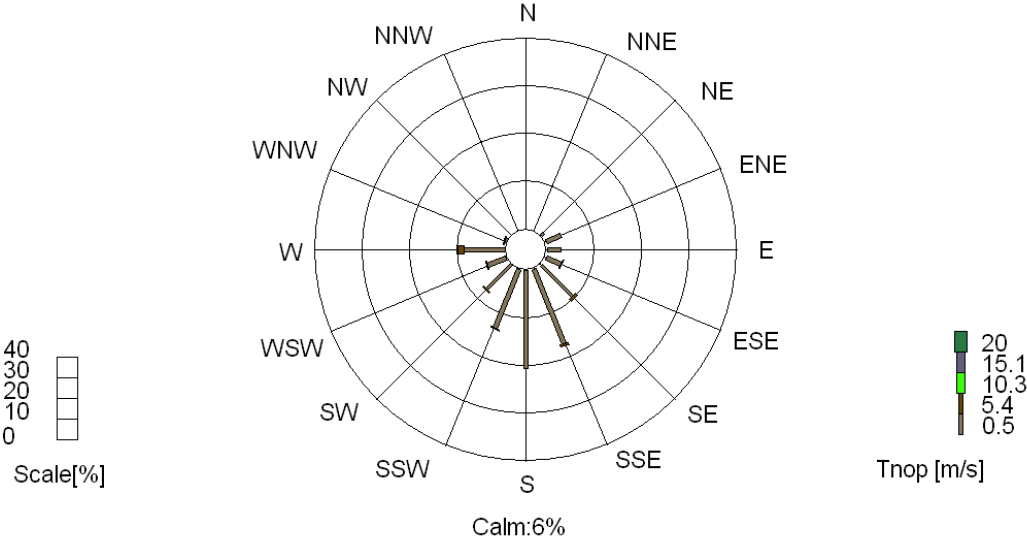
Monthly Wind Rose Terveyskeskus joulukuu 2011 Station:Terveyskeskus Avg:1 Hour
