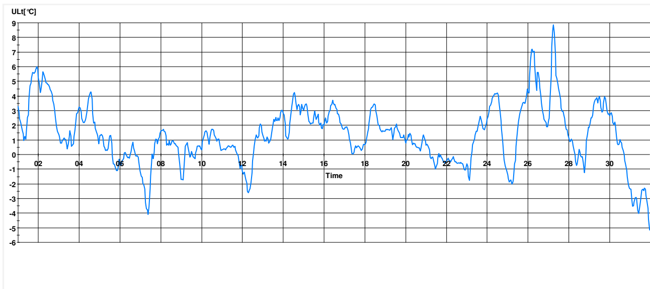
ULt[°C] Monthly Report Terveyskeskus 12.2011 Interval 1 Hour
